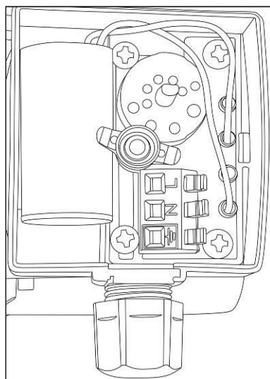
Рис. 5 Клеммы для подключения кабеля
